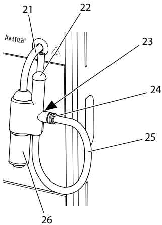
Kuva 4: Cappuccinator
