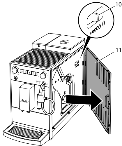
Obr. 14: Nastavení stupně mletí
