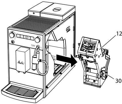
Kuva 16: Suodatusyksikön irrottaminen
